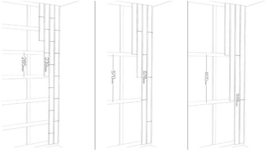
Tiles by Thermory -paneelien asennus pystysuoraan
