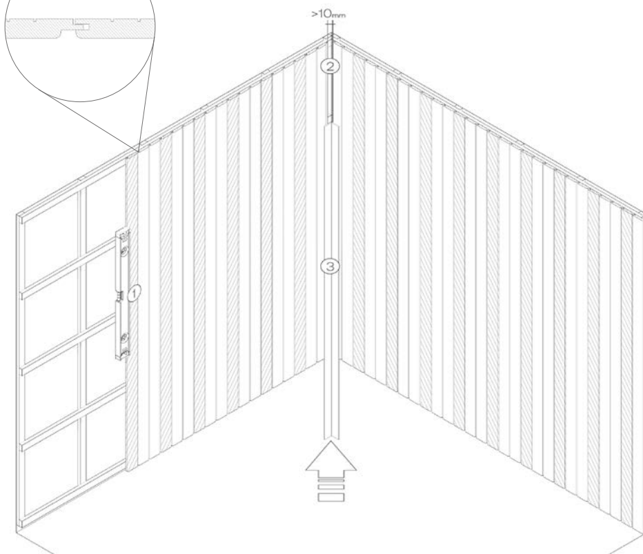
Seinäpaneelien asennus pystysuoraan
