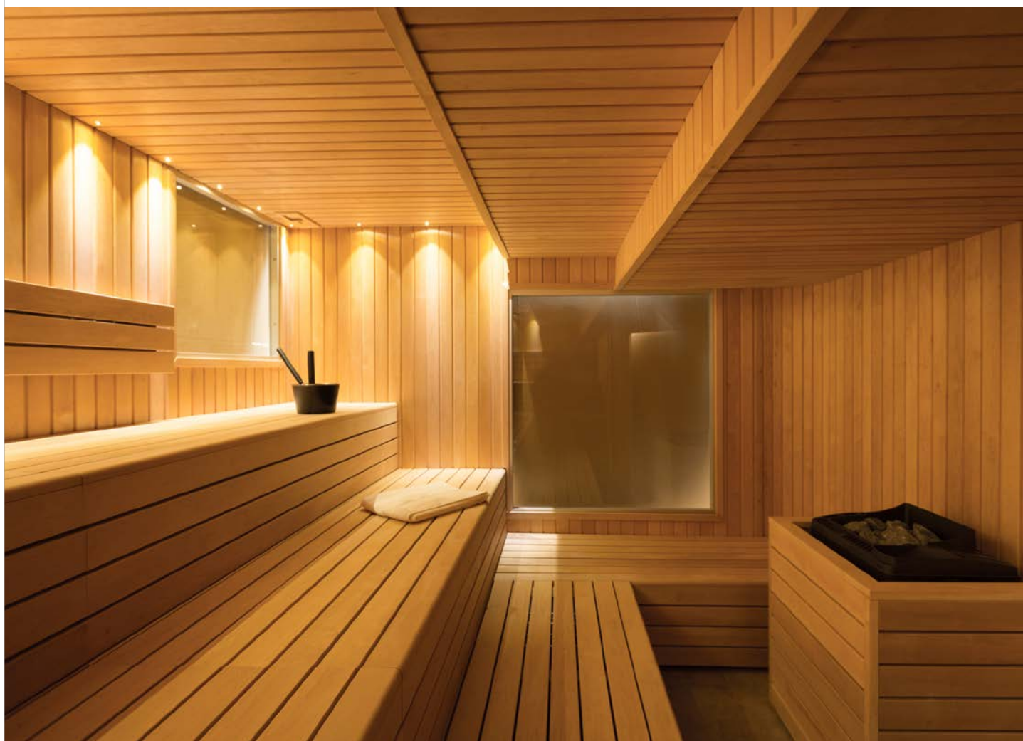
Seinäpaneelit: STP 15x90 leppä, laudelaudat: SHP 28x90 leppä. Spa-sauna Saksassa.
